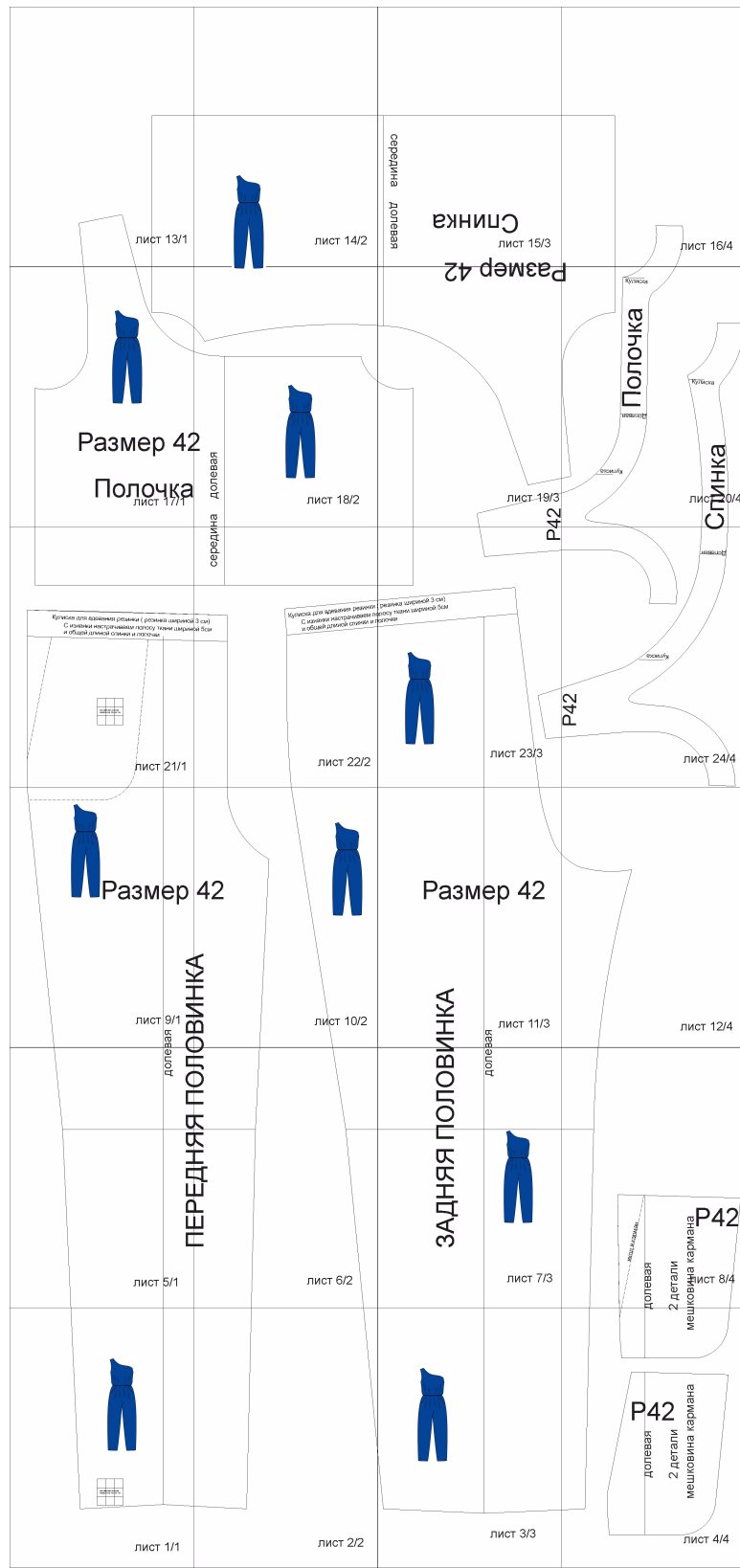
Схема выкройки
